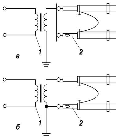
Рисунок 1 – Принципиальные схемы испытания указателя напряжения для проверки совпадения фаз по схеме согласного (а) и встречного (б) включения
